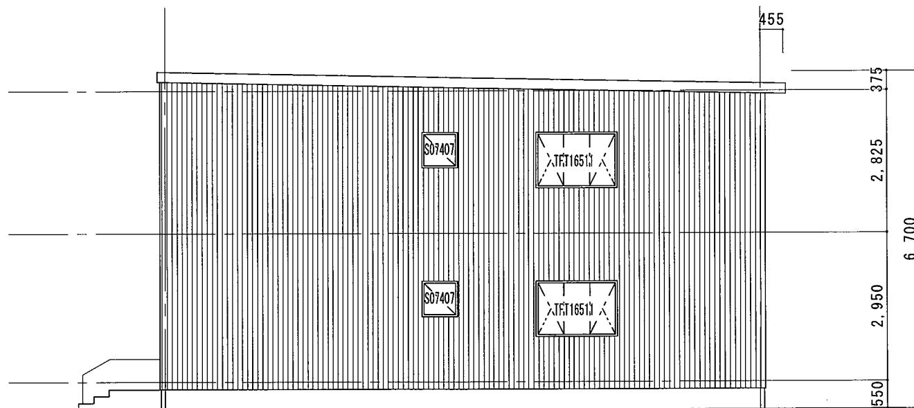
南立面图
