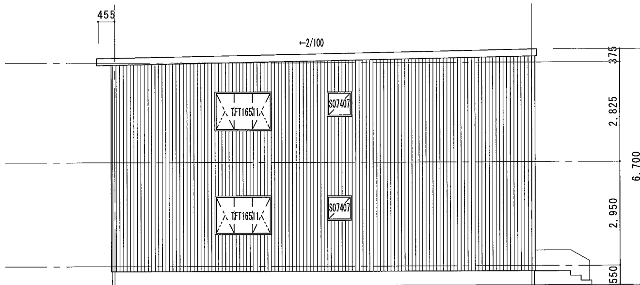
北立面图
