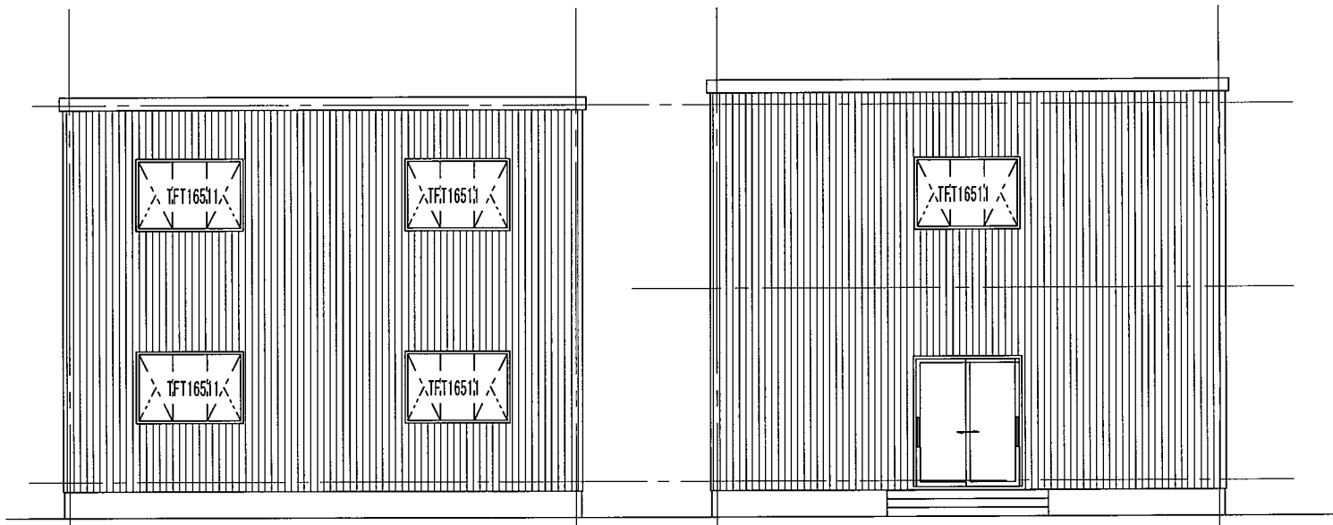
西立面图
